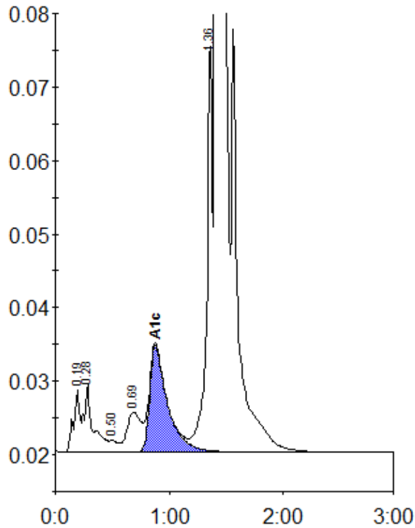
Peak table - ID: 10460772
